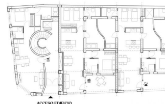
PLANTA I
