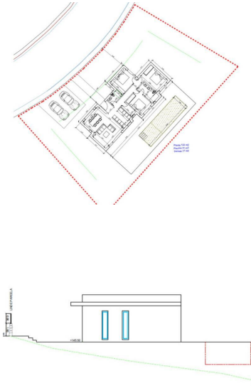
ALZADO SUROESTE
