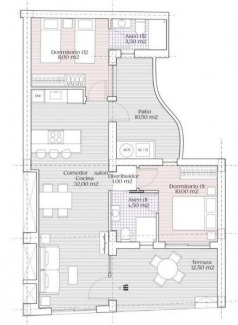
PLANTA I
