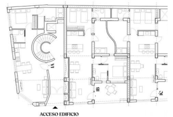
PLANTA I
