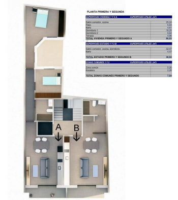
Planta Primera y segunda. Estudio B y Vivienda A
