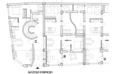
PLANTA 1
