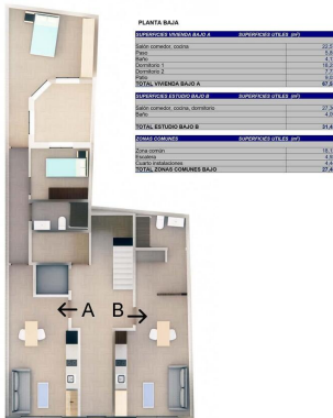
Planta Baja. Estudio B y Vivienda A
