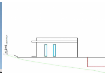
ALZADO SUROESTE
