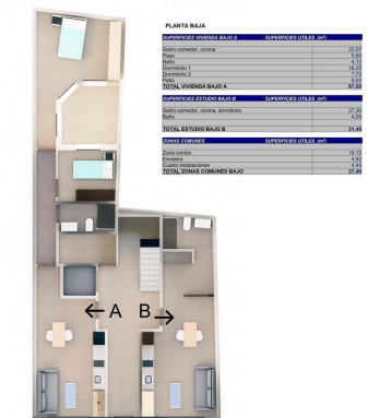
Planta Baja. Estudio B y Vivienda A
